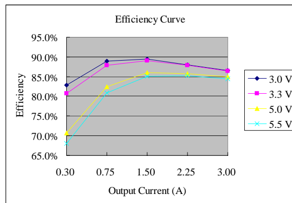
Vo=1.5 V
