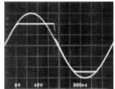
A_V = -1 , V_{IN} = 12V_{p-p} 1190 G24
