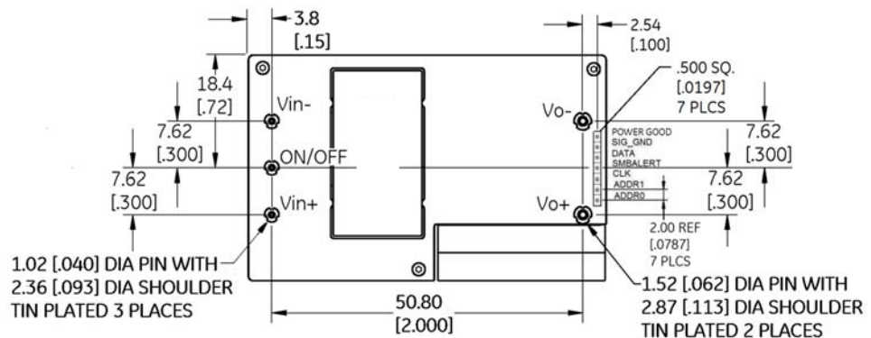
BOTTOM VIEW***
